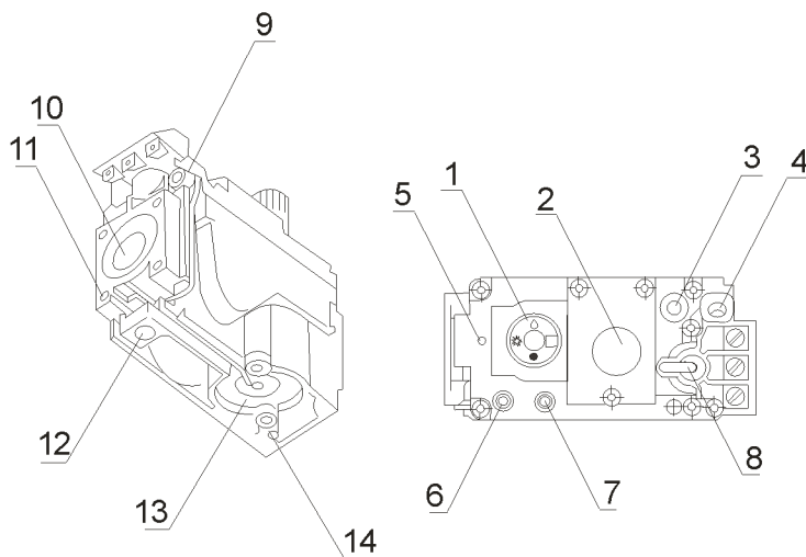
Рис. 3-3. Автоматика безопасности «SIT 820 NOVA»
