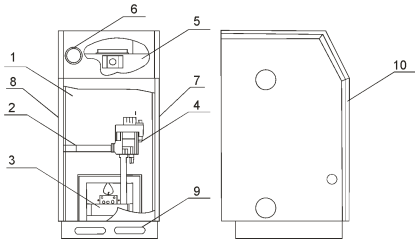
Рис. 2-1. Газовый напольный котел ARIDEYA с авт. «630 EUROSIT»
