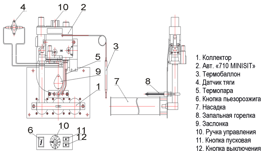
Рис. 3-2. Автоматика безопасности «710 MINISIT»
