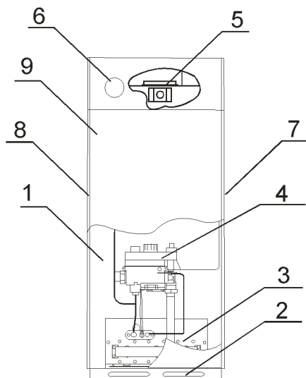
Рис. 2-3. Газовый напольный котел ARIDEYA с авт. «710 MINISIT»
