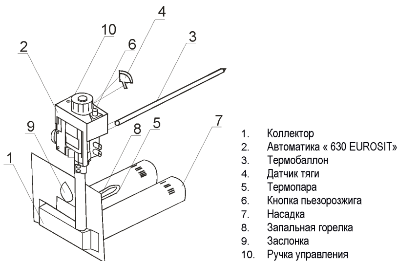
Рис. 3-1. Автоматика безопасности «630 EUROSIT»
