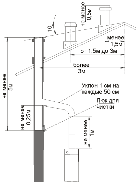
Рис.4-2. Примерная схема монтажа котла в открытой системе отопления.
